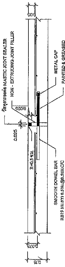
รายละเอียด EXPANSION JOINT (ทุกระยะไม่เกิน 30 เมตร) NOT TO SCALE
