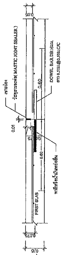
รายละเอียด CONTRACTION JOINT (ทุกระยะไม่เกิน 10 เมตร) NOT TO SCALE
